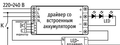
Схема подключения БАП в светильнике DPO-МС1-А
